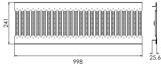
2А995924 Решетка водоприёмная Ecotekc STANDART 200 стальная штампованная оцинкованная кл. А15
