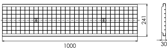
2А995929 Решетка водоприёмная Ecotekc STANDART 200 чугунная щелевая кл. С250
