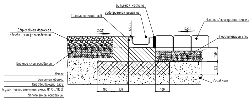
Схема монтажа водоотводного лотка Ecotek STANDART 100.65 H 69 в поверхность, мощеную штучным камнем и асфальтобетонным покрытием. Класс нагрузки C 250 .
